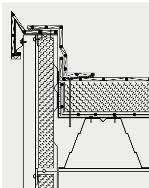
Attikaabschluss mit Verbundblech- Organgprofil
