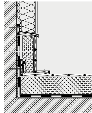
Wandanschluss gedämmt mit Z-Profil
