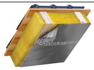
Abb. 4: Einsatz von innen
