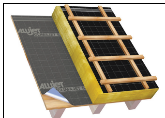
Abb. 3: Einsatz unter Aufdachdämmung
